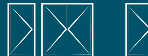
Porte-fenêtre 1 et 2 vantaux avec seuil
